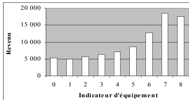
Figure 6. Revenu journalier moyen des ménages selon l'indicateur d'équipement* * voir figure 2 pour les variables entrant dans la composition
